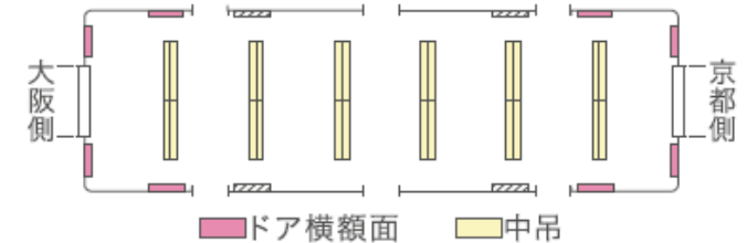
3000系車内図面
